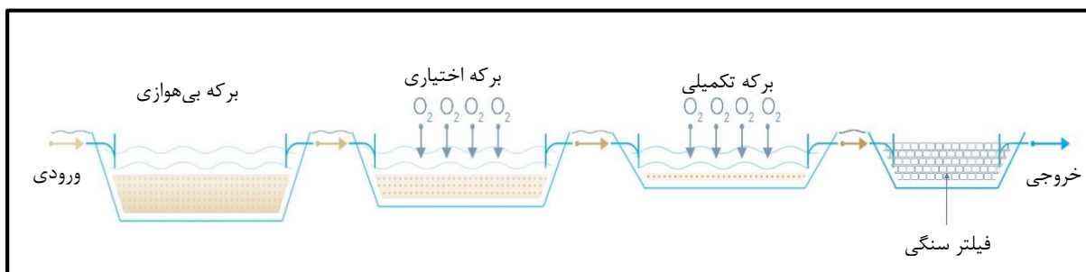
شکل ۷-۲۱- فیلتر سنگی
