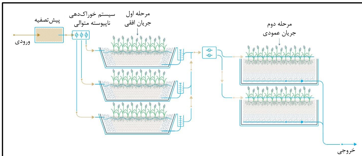
شکل ۷-۱۰- وتلندهای ساخته شده چندگانه (هیبریدی)
