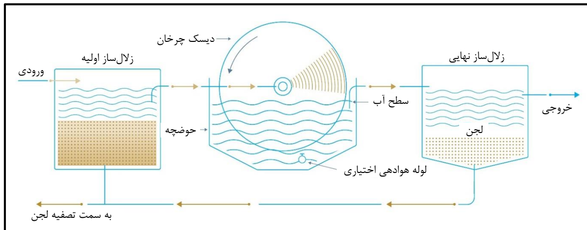
شکل ۷-۱۵- تماس دهنده‌های بیولوژیکی چرخان
