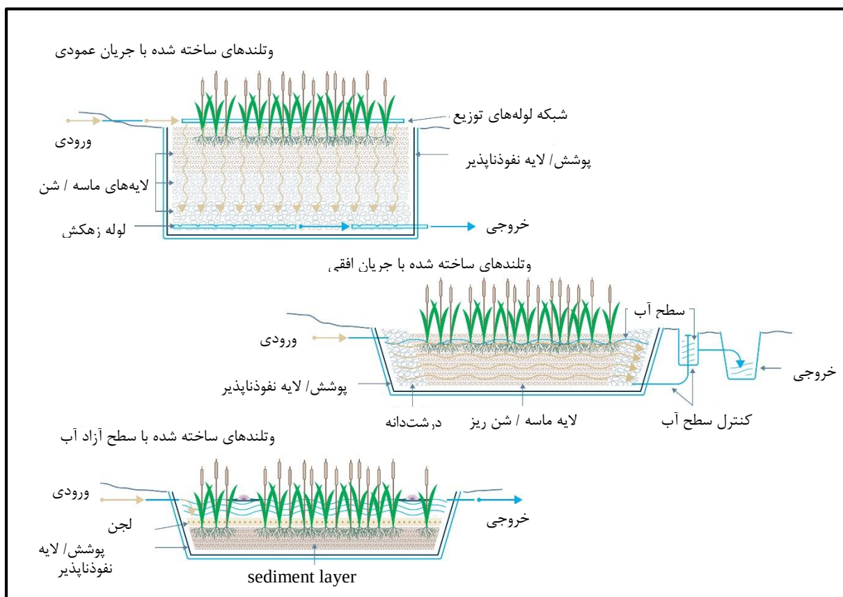
شکل ۷-۹- و تلندهای ساخته شده یک مرحله‌ای
