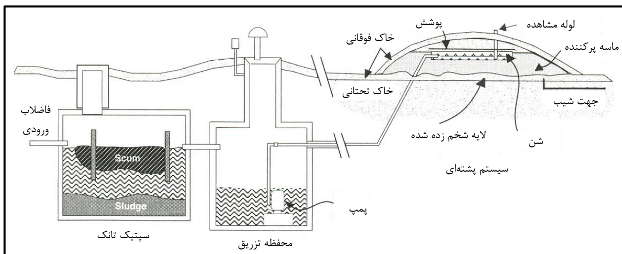
شکل ۹-۴- سامانه تصفیه فاضلاب به روش پشته‌ای
