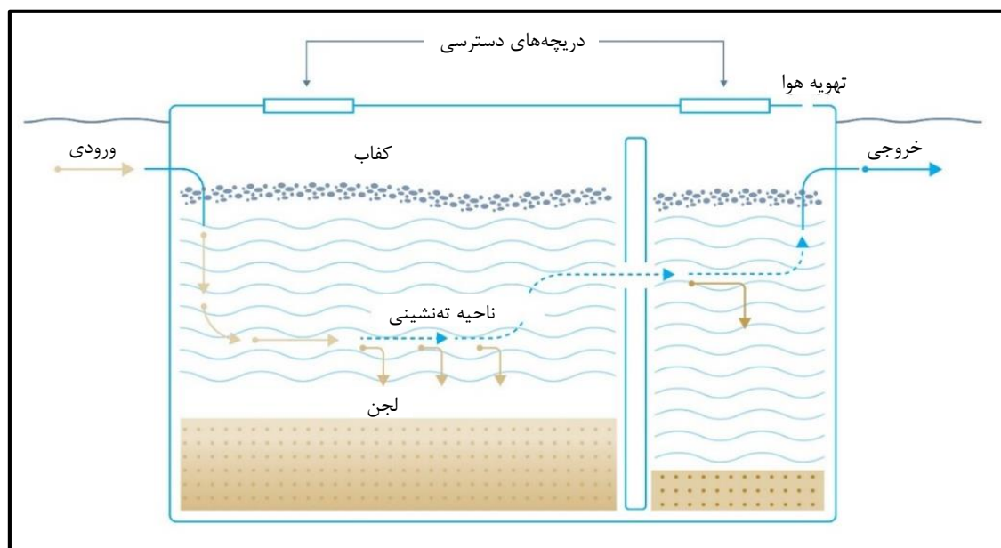
شکل ۷-۱- سپتیک تانک
