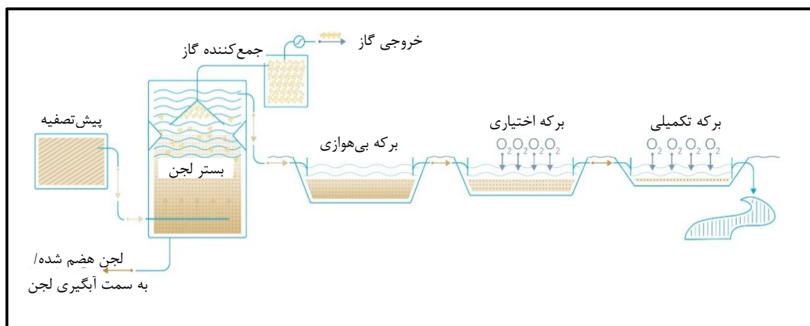
شکل ۷-۱۶- سامانه UASB به همراه برکه تثبیت فاضلاب
