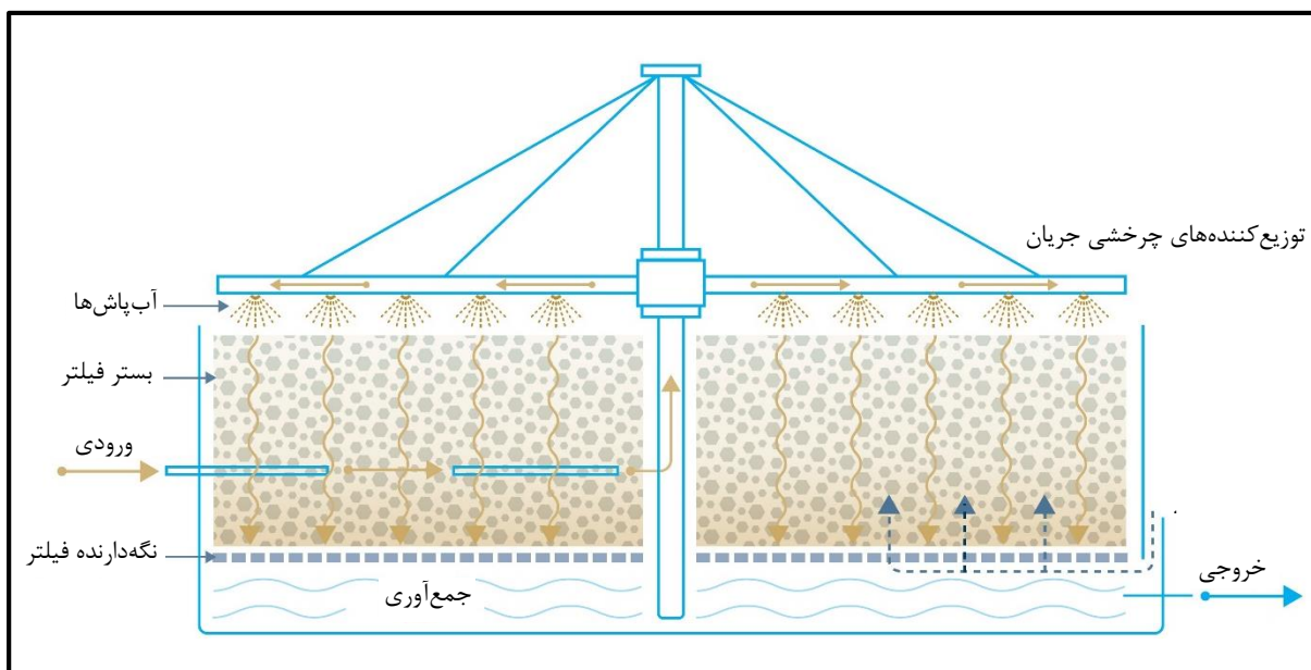
شکل ۷-۱۴- صافی چکنده
