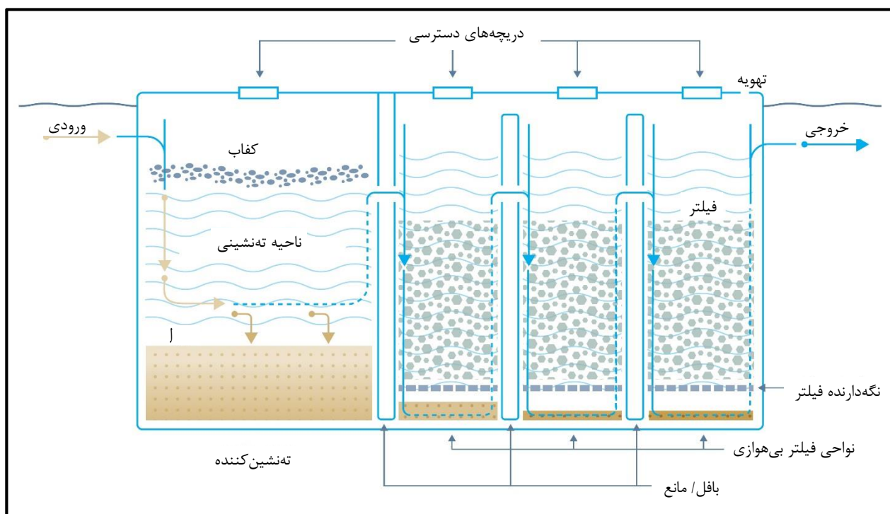
شکل ۷-۵- فیلترهای بی‌هوای
