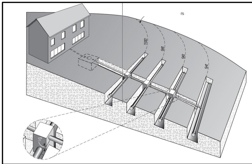
شکل ۹-۱- نمای شماتیک سامانه‌های دفع پلکانی
