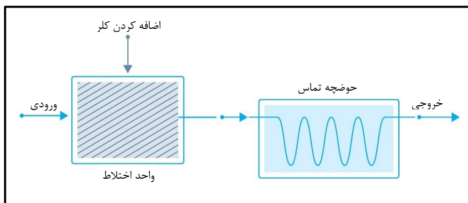
شکل ۷-۱۹- گندزدایی با کلر
