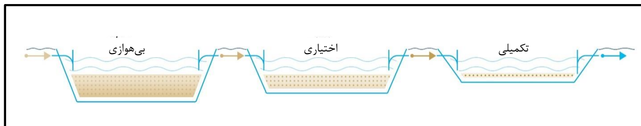
شکل ۷-۶ - برکه‌های تثبیت فاضلاب
