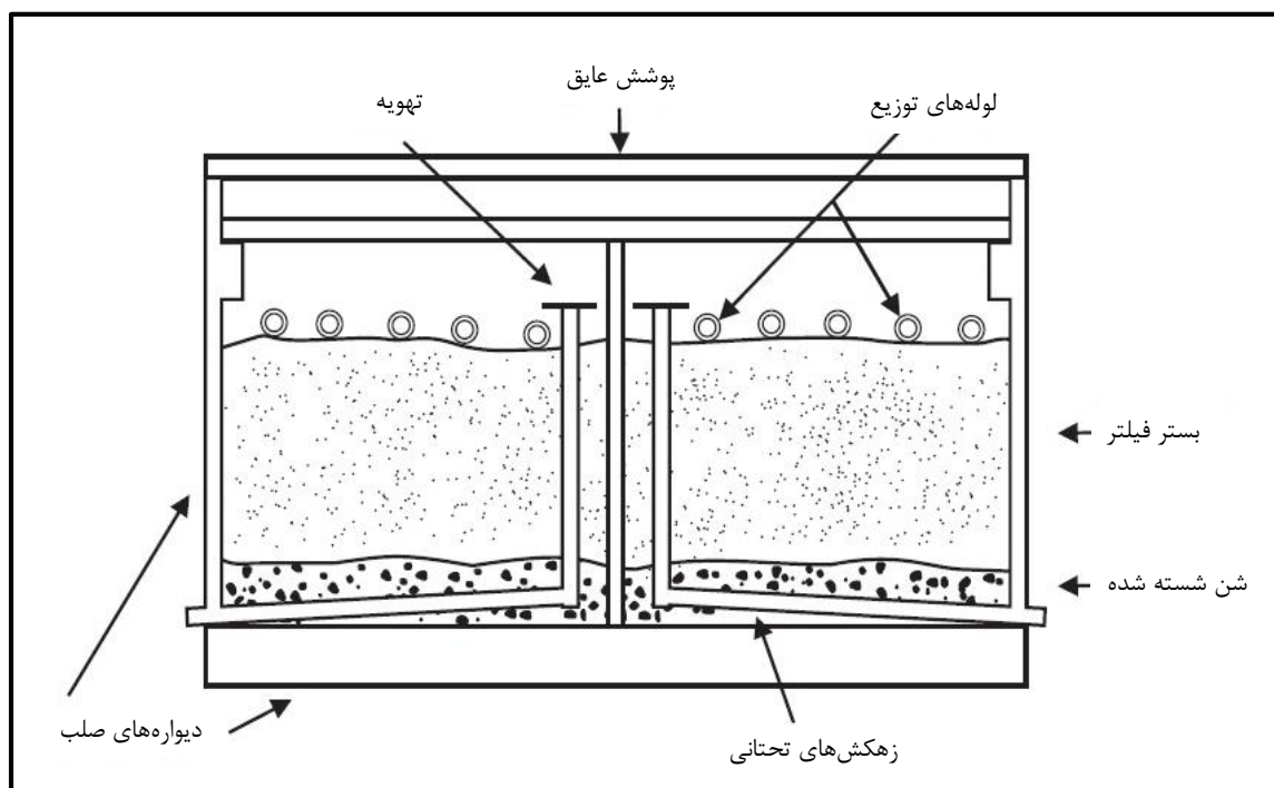
شکل ۹-۲- نمای شماتیک فیلتر ماسه‌ای متناوب - نوبه‌ای
