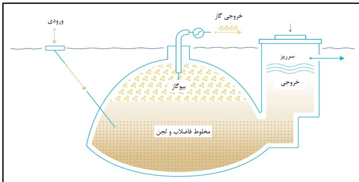
شکل ۷-۲- هاضم بیوگاز
