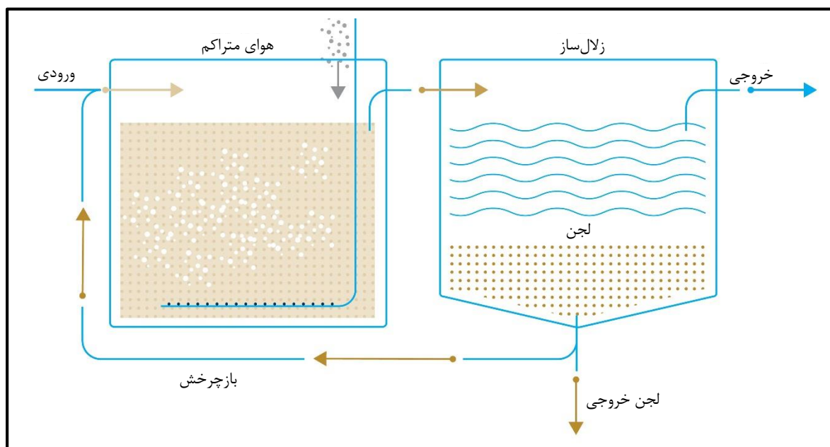
شکل ۸-۱۲- لجن فعال - هوادهی گسترده
