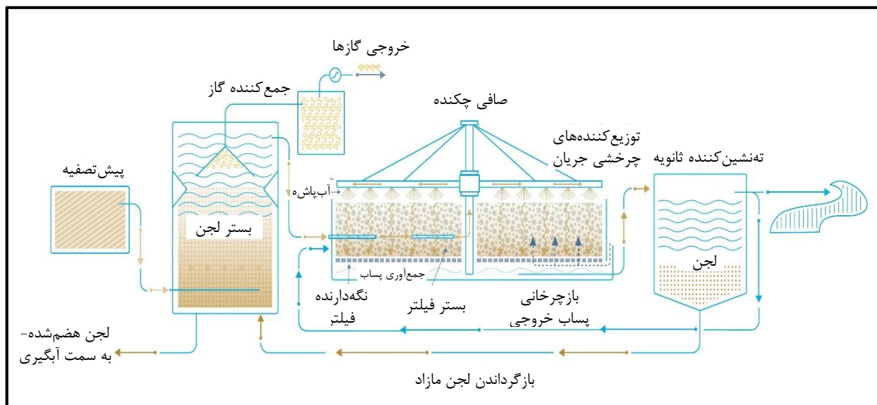
شکل ۷-۱۷- سامانه UASB به همراه صافی چکنده
