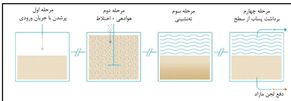
شکل ۷-۱۳- رآکتور ناپیوسته متوالی
