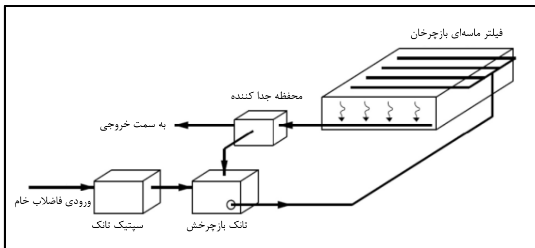
شکل ۹-۳- شمای فیلتر ماسه‌ای متوالی با بازچرخش
