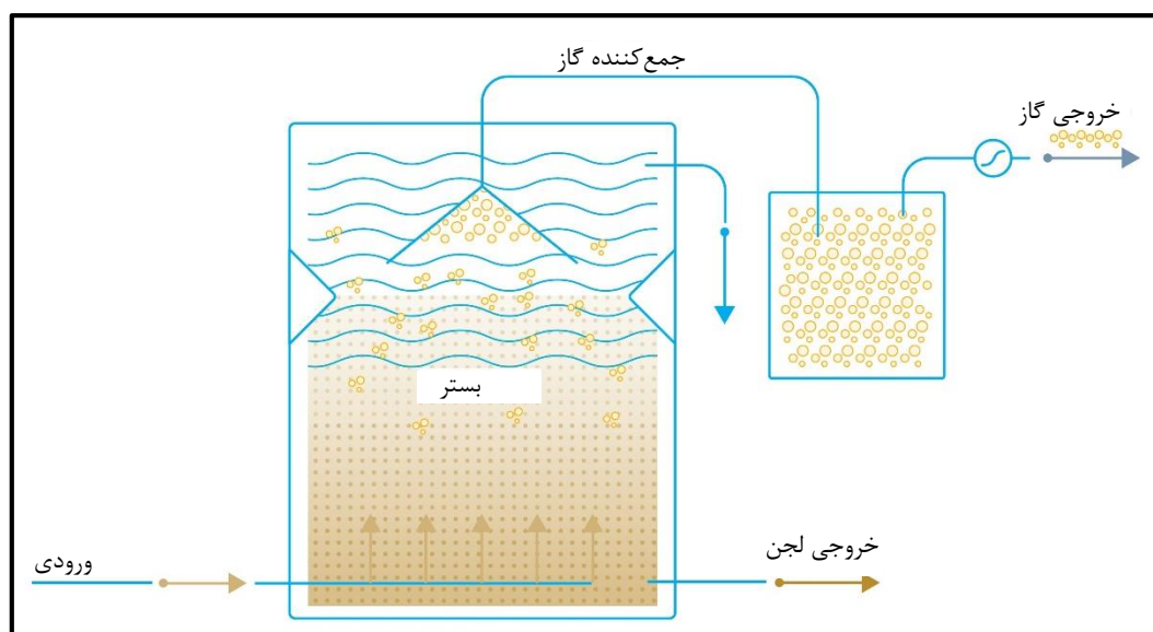
شکل ۷-۱۱- راکتور بستر بی‌هوازی لجن با جریان رو به بالا
