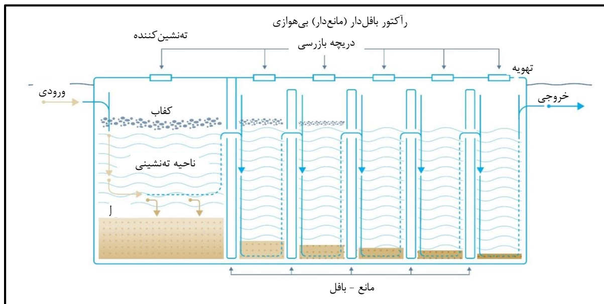
شکل ۷-۴- راکتور بافل‌دار (مانع‌دار) بی‌هوازی
