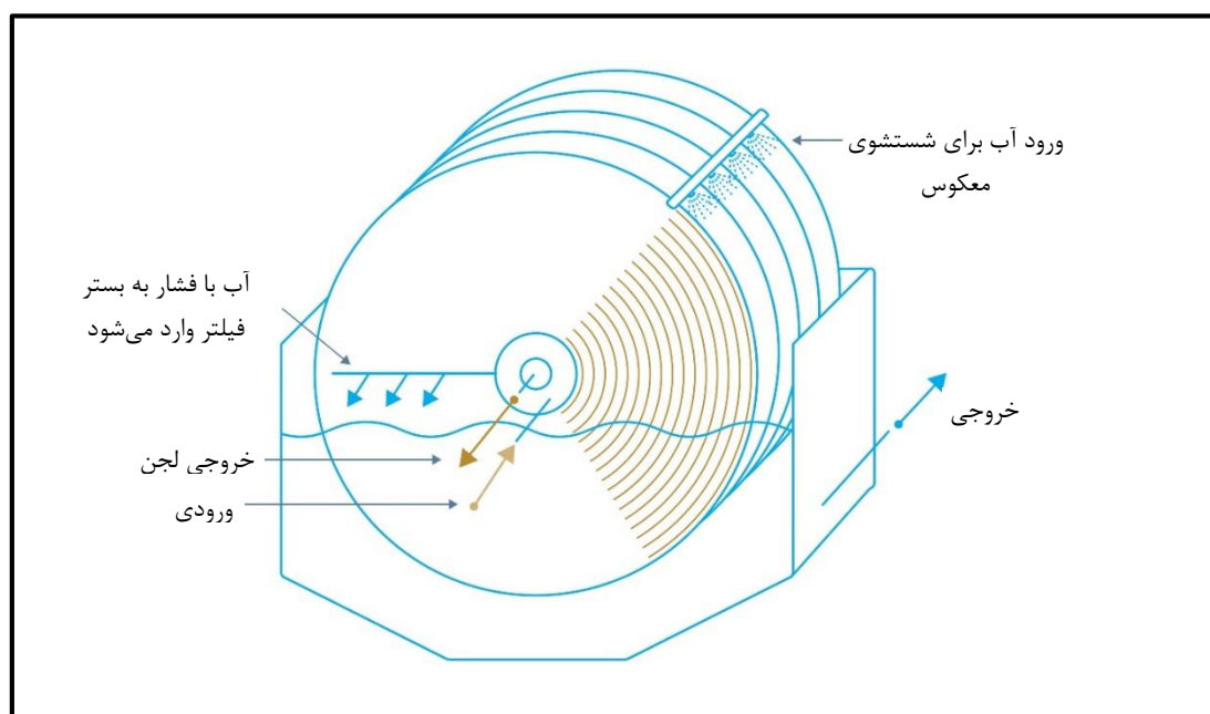
شکل ۷-۲۲- فیلتر چرخان دیسکی
