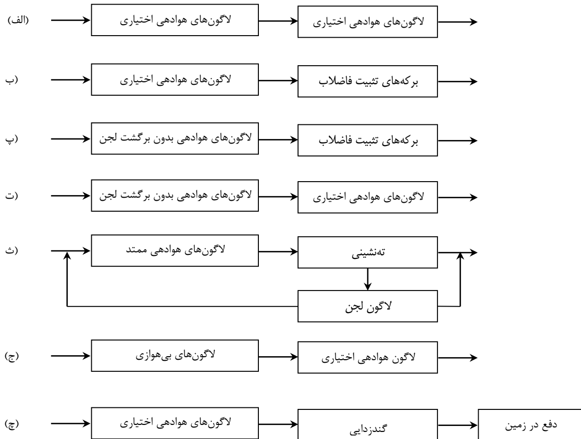
شکل ۷-۸- طرح‌های مختلف برکه و لاگون
