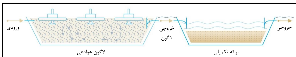
شکل ۷-۲۰- برکه‌های تکمیلی
